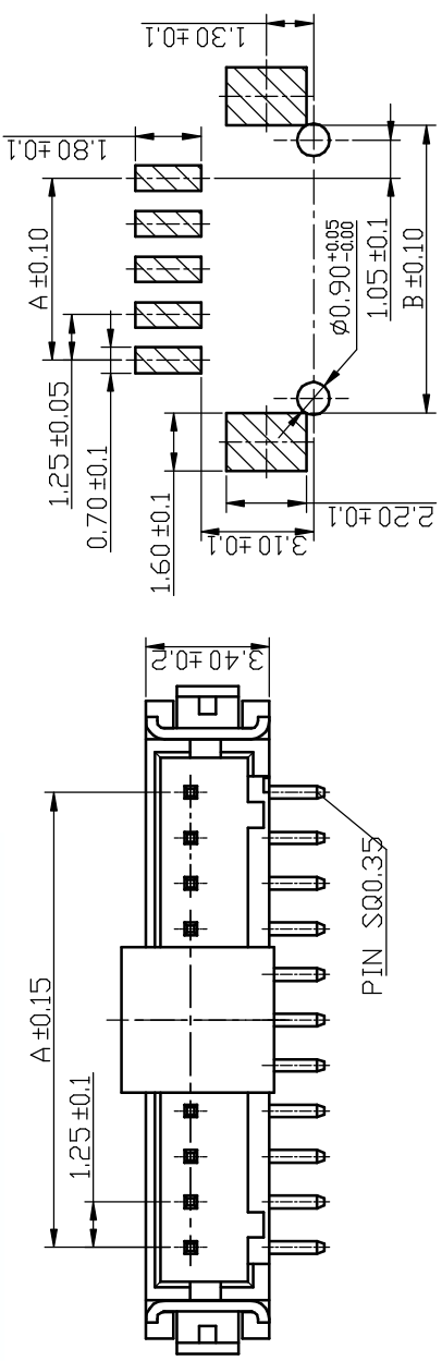
P.C.B LAYOUT
