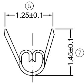
A-A SEC
